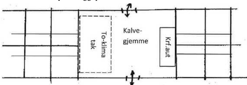
Illustrasjonen viser hvordan et kalvegjemme kan innpasses inn i dobbeltraden i et fjøs med dobbel liggebåsråd. Toklimataket kan vippes opp for lettere reinhold. Denne bingeløsningen kan også brukes som kalvingsbinge.
