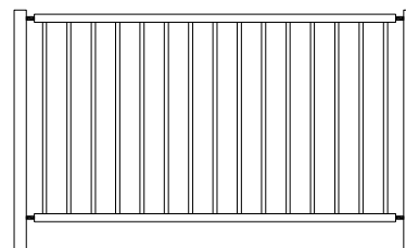
Skille - vertikale rør
